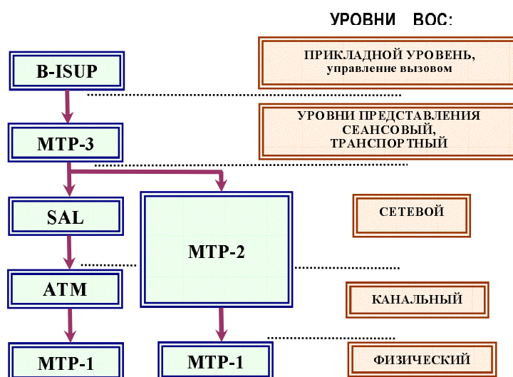
Рис. 1.20. Стек протоколов при использовании подсистемы В-ISUP
