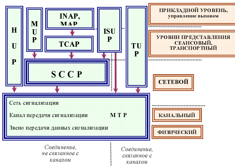
Рис. 1.4. Соответствие архитектуры ОКС № 7 и уровней модели ВОС.
