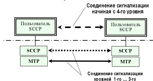
Рис. 1.18. Соединение сигнализации
