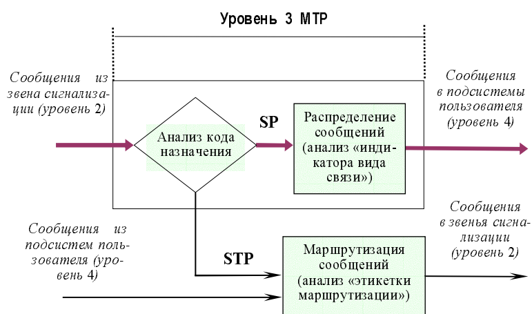
Рис. 1.17. Функции обработки сообщений на уровне 3 МТР
