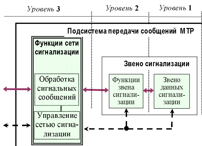
Рис. 1.15. Общая структура подсистемы МТР: ← → - поток сигнальных сообщений, ← → - управление и индикация
