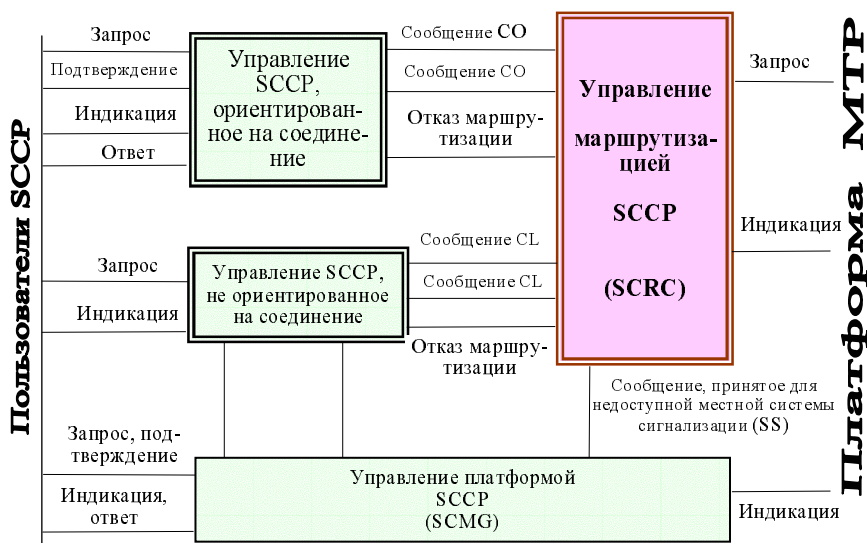
Рис. 1.19. Структура SCCP
