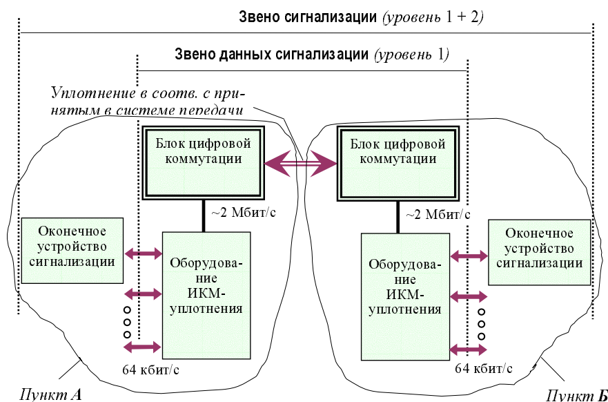
Рис. 1.16. Конфигурация звена данных сигнализации
