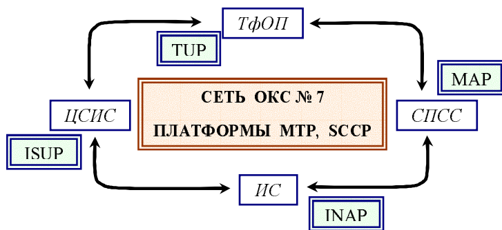
Рис. 1.3. Взаимодействие цифровых сетей по протоколам ОКС № 7
