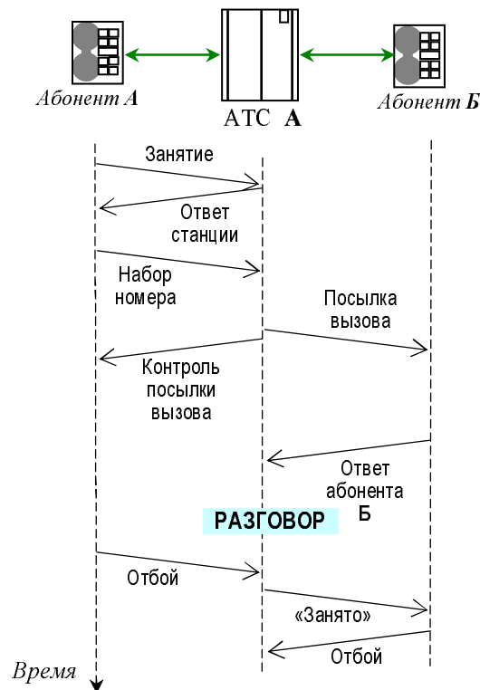
Рис. 1.2. Пример абонентской сигнализации
